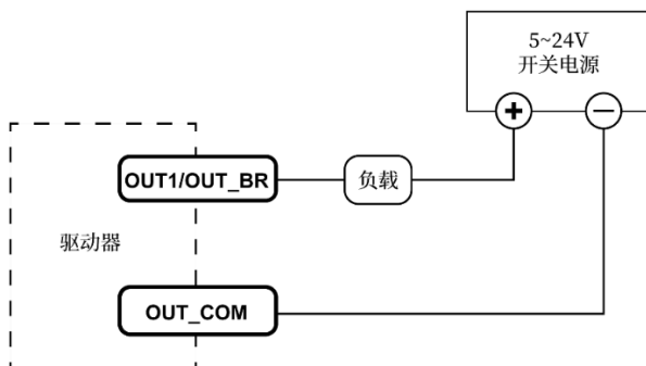
输出信号灌电流输出的连接方式
