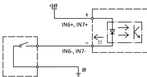
NPN 输入示意图
